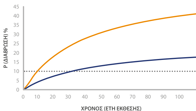
ΠΙΘΑΝΟΤΗΤΑ ΔΙΑΒΡΩΣΗΣ – ΕΠΙΚΑΛΥΨΗ ΣΚΥΡΟΔΕΜΑΤΟΣ = 50 MM
