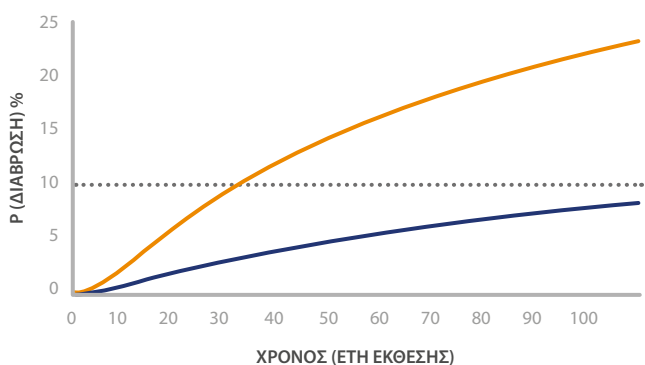
ΠΙΘΑΝΟΤΗΤΑ ΔΙΑΒΡΩΣΗΣ – ΕΠΙΚΑΛΥΨΗ ΣΚΥΡΟΔΕΜΑΤΟΣ = 65 MM
